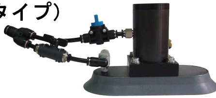
写真左は90x190長円形パッド。右はφ120円形パッド。
