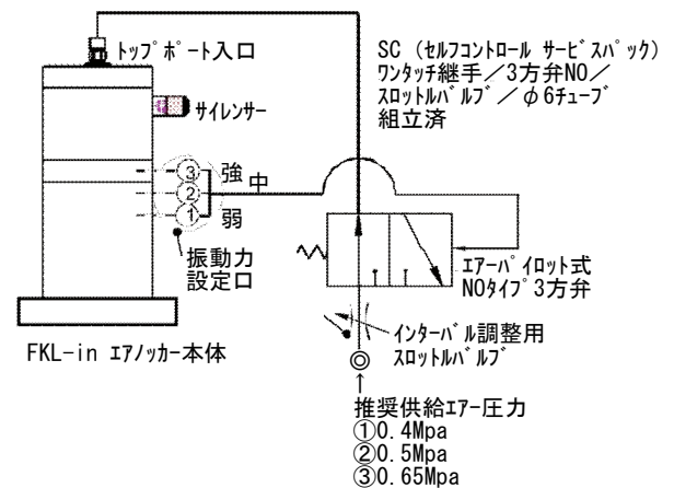
インターバルパケットモード時の配管例 （納入時は振動力の設定は「中」②が標準です）
