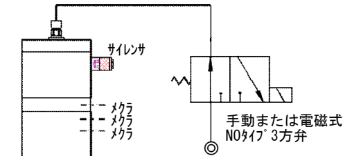
FKL-in エアノッカー本体のみ
