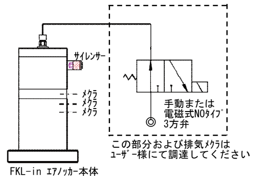
シングルパケットモード時（ユーザーオプション）の配管例 （排気ポート①②③はすべてメクラにしてください）
